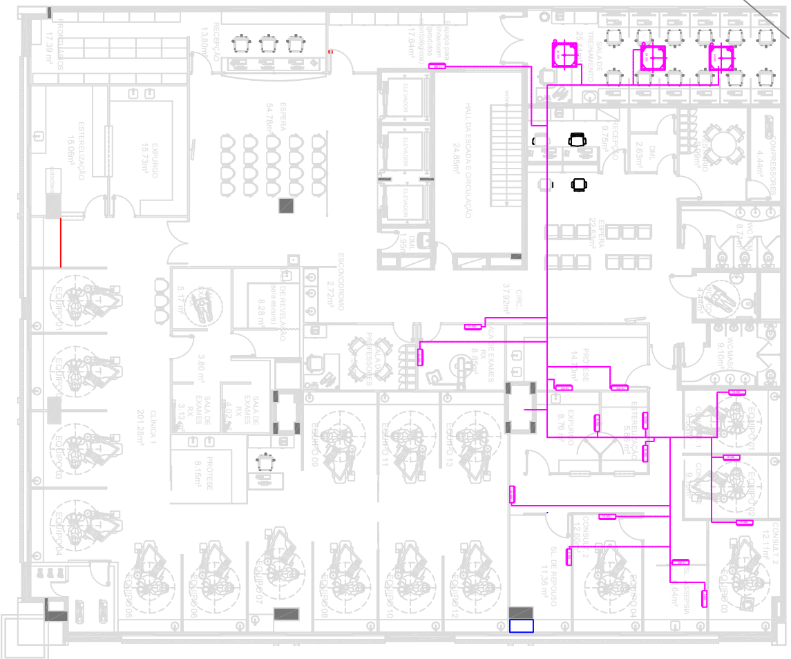
01 PLANTA DE LOCAÇÃO DAS EQUIPAMENTOS - AR-CONDICIONADO
