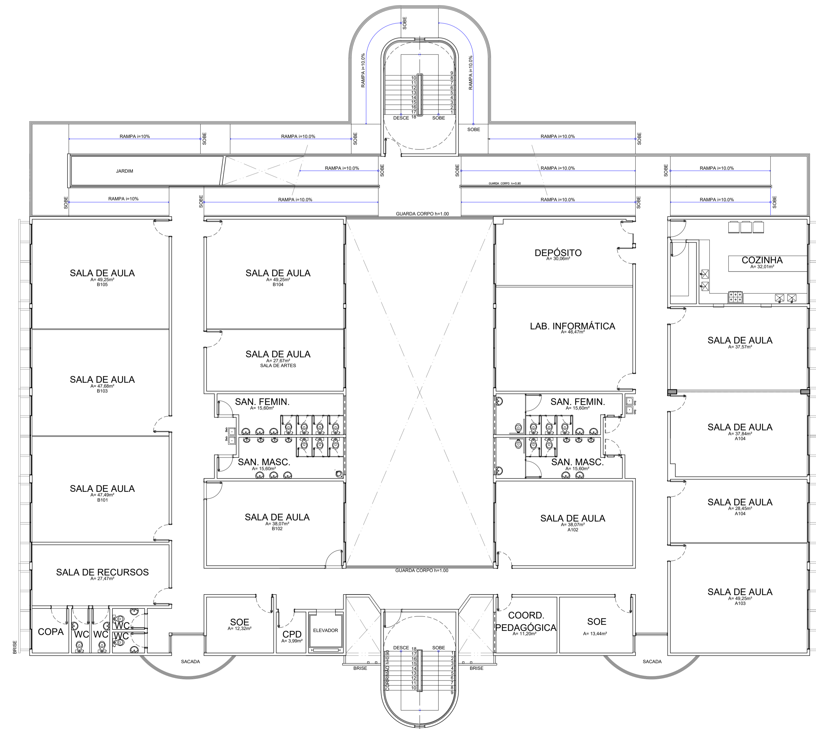
03 PLANTA BAIXA - PRIMEIRO PAVIMENTO Etc.: 1/125
