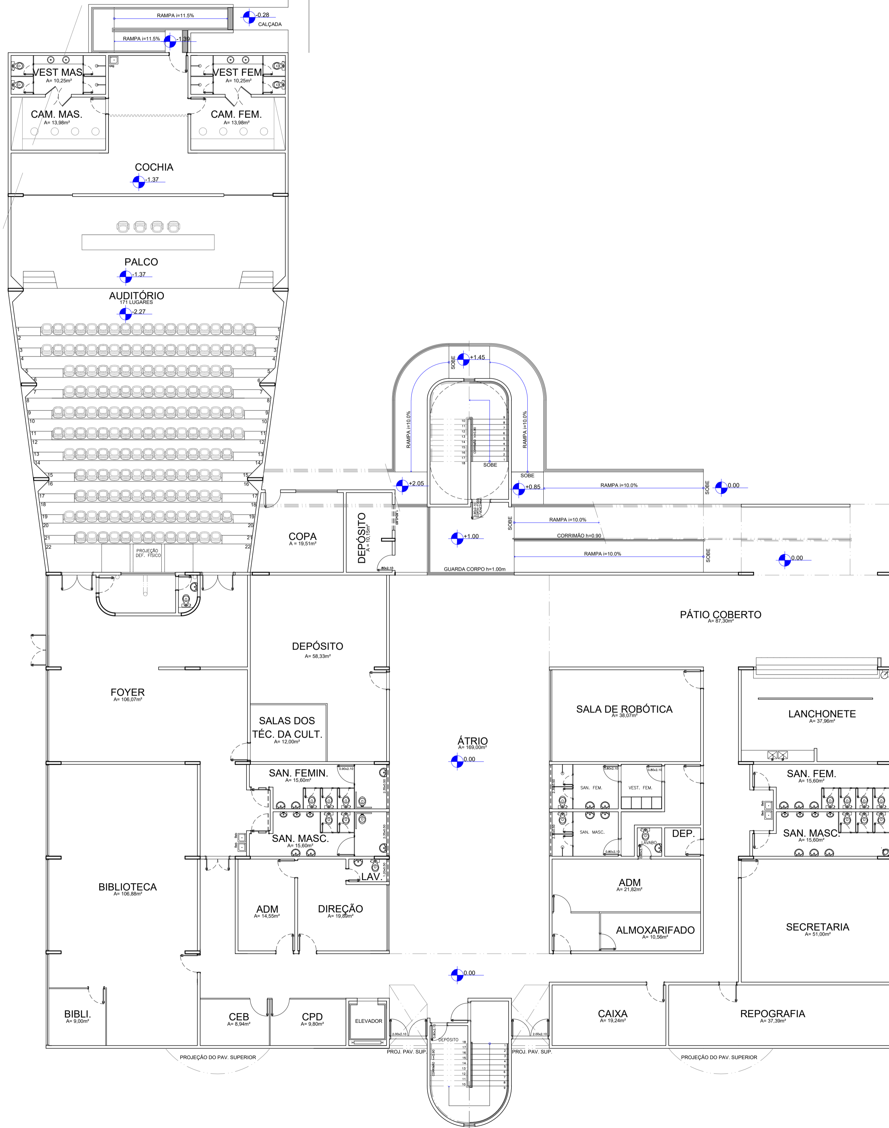
02 PLANTA BAIXA - TÉRREO Etc.: 1/125
