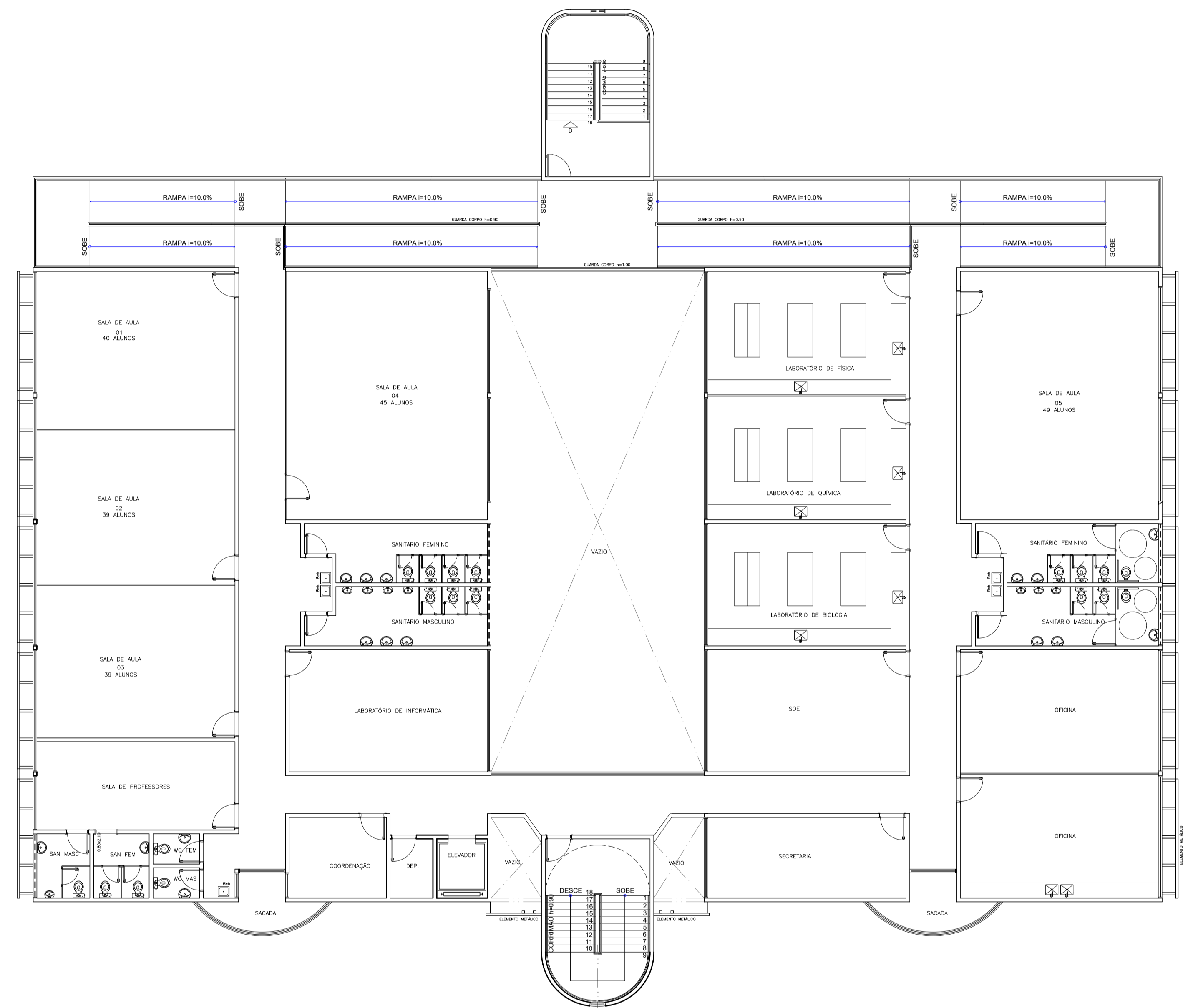
05 PLANTA BAIXA - TERCEIRO PAVIMENTO Esc: 1/125
