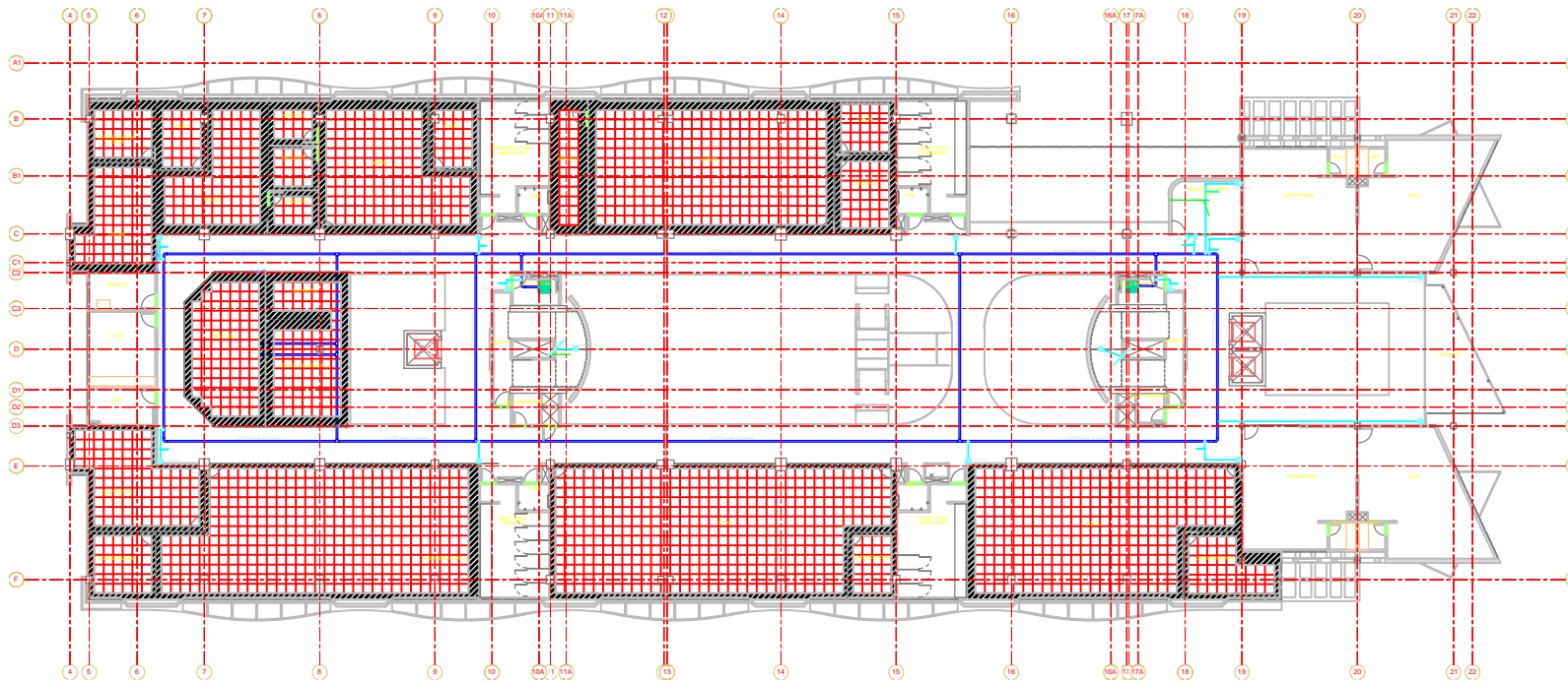
2º PAVIMENTO 1:75
